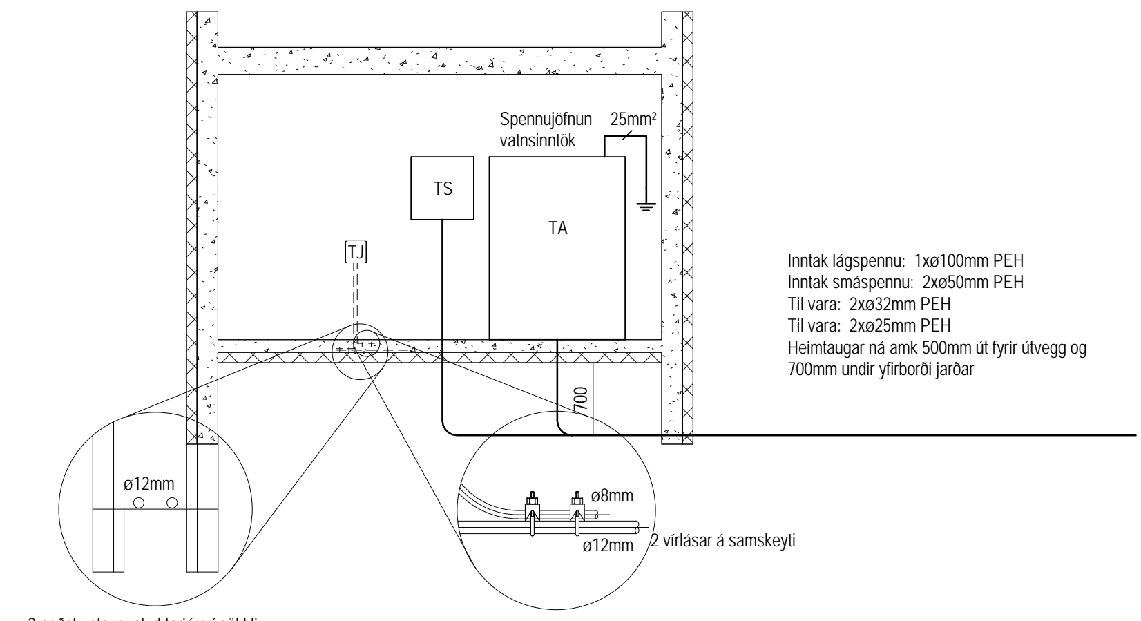
Snið í tæknirými 1 : 50
